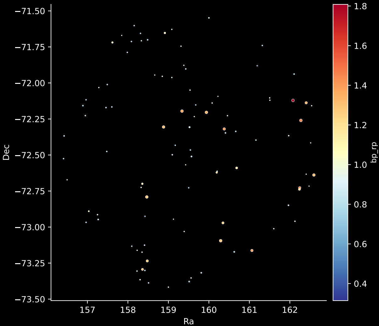
GALAH DR4 Field: [7243] Stars: 98
