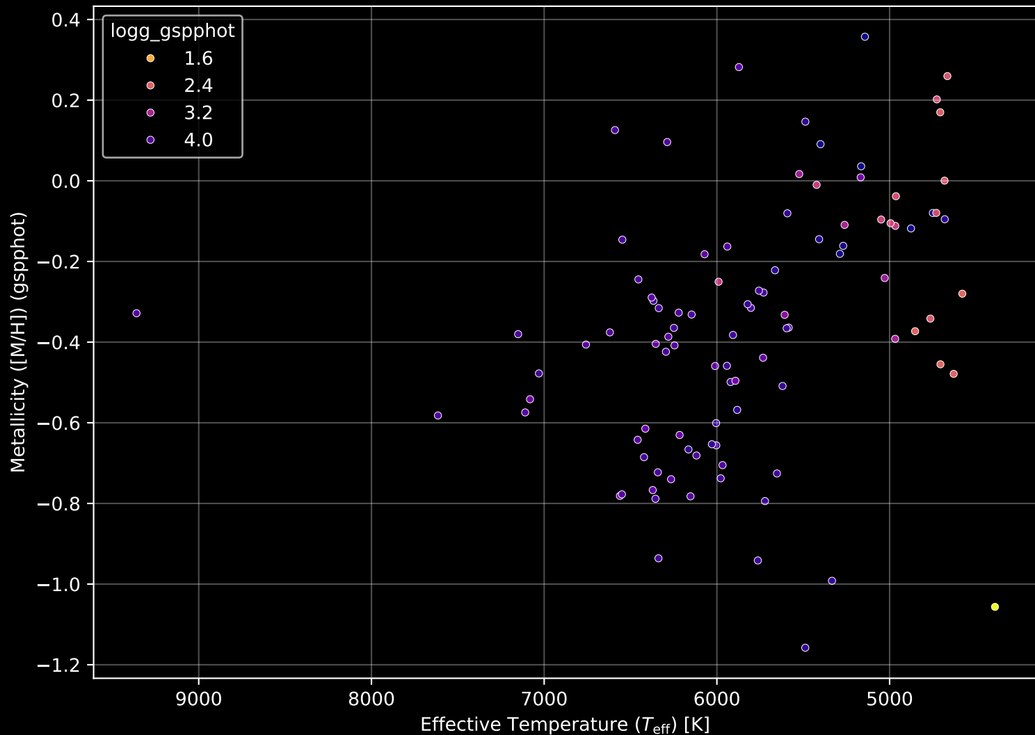
GALAH DR4 Field: [7243] Stellar Population Parameters (n= 98)
